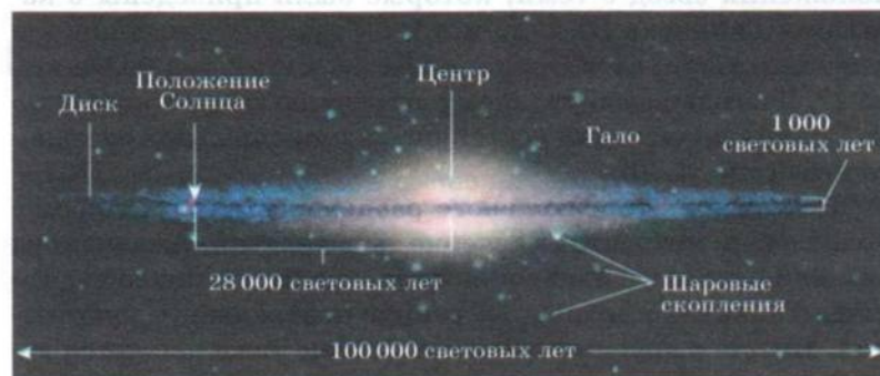
Строение нашей Галактики и положение Солнечной системы: а — схематическое представление; б — фотография
