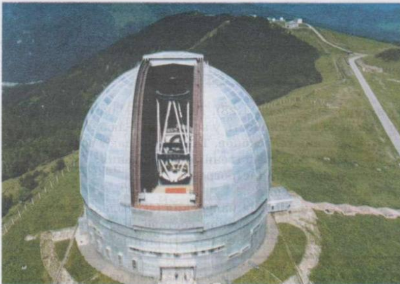
Большой телескоп азимутальный Специальной астрофизической обсерватории Российской академии наук (БТА САО РАН)
