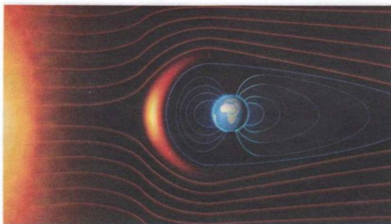
СОЛНЕЧНАЯ СИСТЕМА
