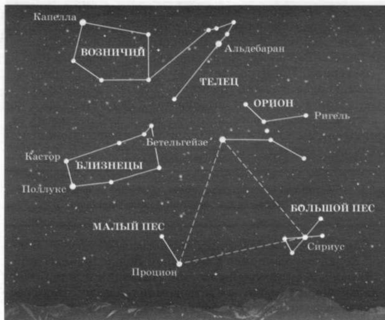
Созвездия зимнего неба
