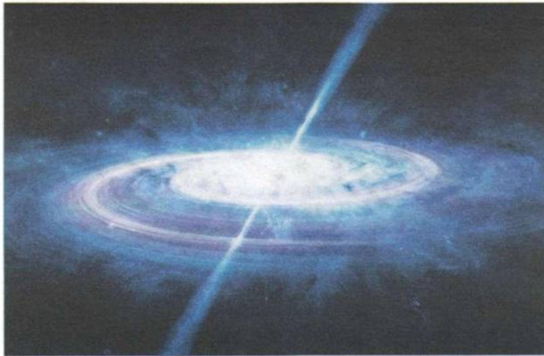
Активное ядро галактики, выбрасывающее газовые струи, — джеты
