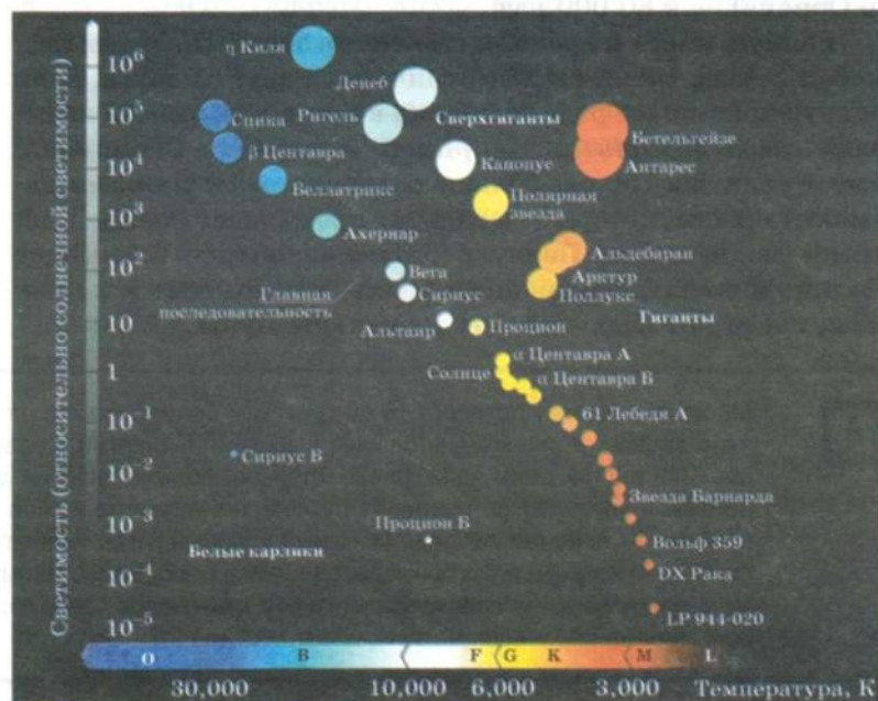
Рис. 3.4 Диаграмма Герцшпрунга—Рассела
