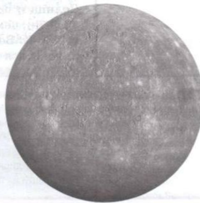
Рис. 2.14 Меркурий
