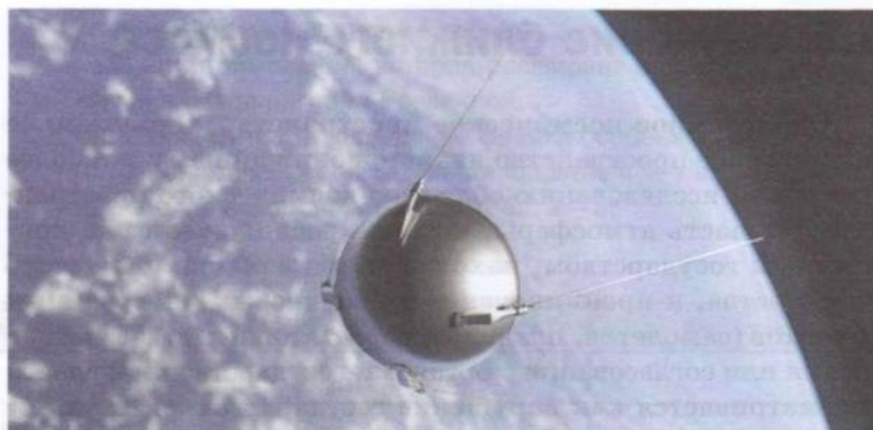
Первый спутник Земли
