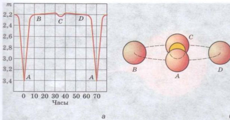
Звезда Алголь ( \beta Персея): а — кривая блеска звезды; б — взаимное расположение элементов этой двойной звездной системы
