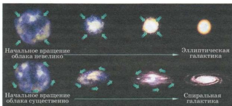
Образование эллиптических и спиральных галактик
