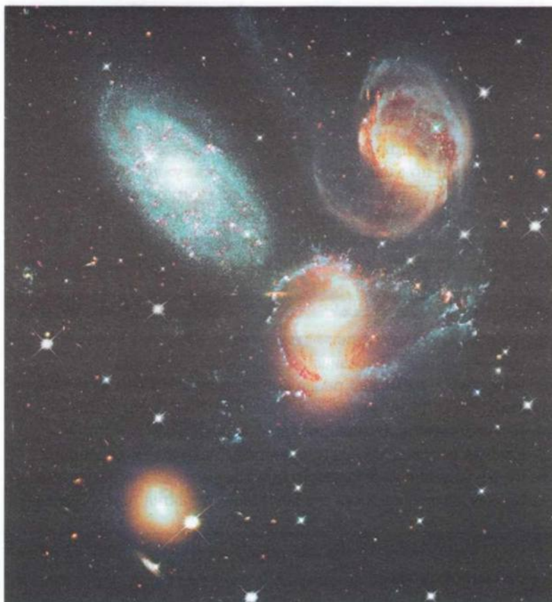
Квинтет Стефана — группа из четырех взаимодействующих галактик
